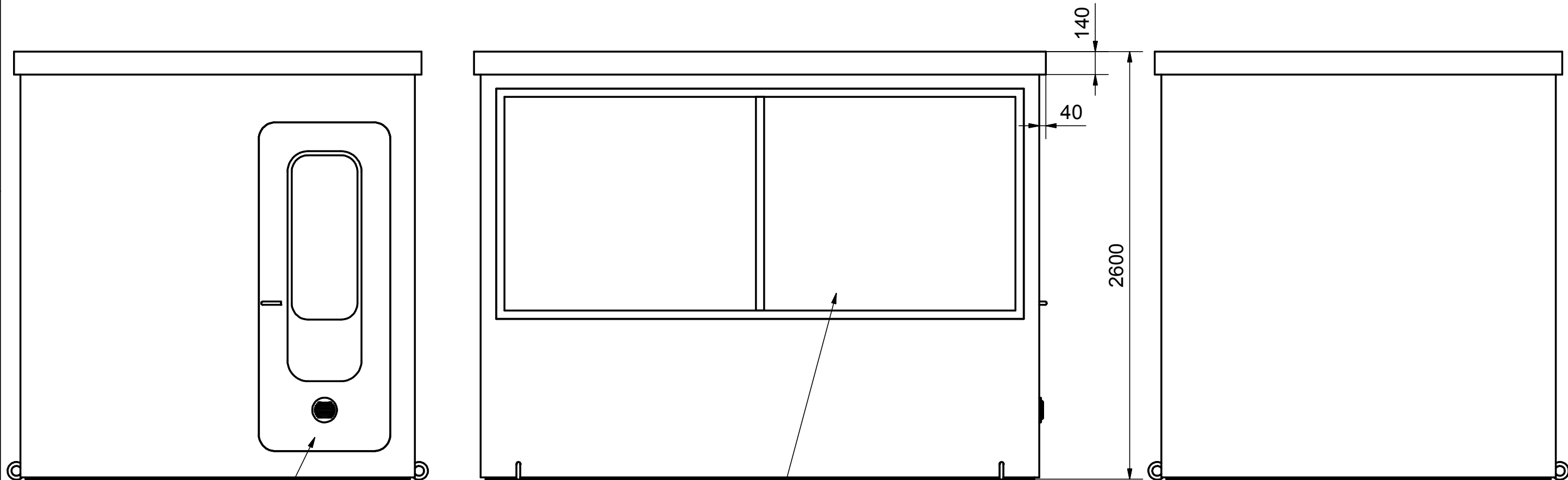
GFK-Türe inkl. Glas ESG
